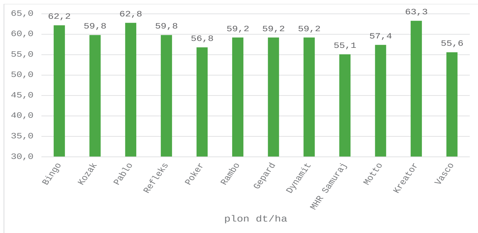
Wykres 1. Plonowanie owsa w doświadczeniach PDO. Rok zbioru: 2024
